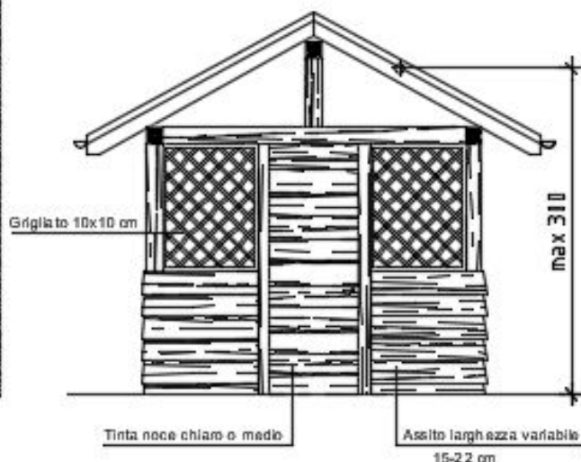
VISTA FRONTALE
